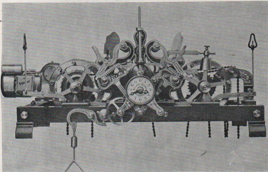
Reloj de remontaje eléctrico, horas y cuartos, con repetición
