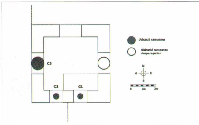
Planta de la sala de campanes.
