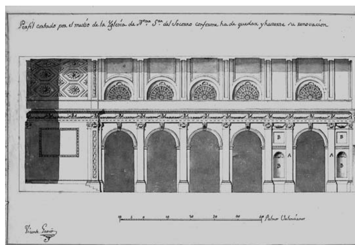
Fig. 14. Perfil con el proyecto de reforma de la iglesia del dicho convento del Socorro por el arquitecto Vicente Gascó.
