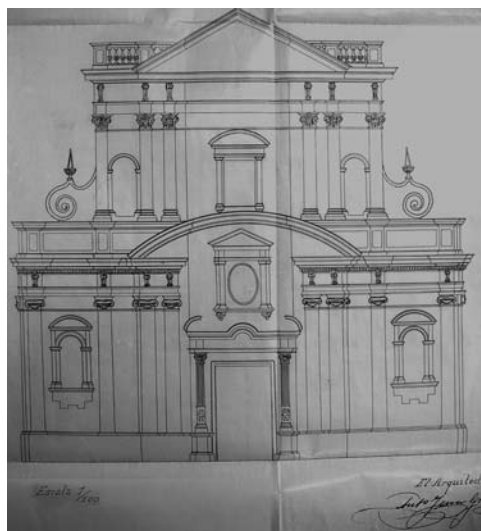
Fig. 4. Alzado de la fachada de la iglesia de la antigua Congregación de San Felipe Neri de Valencia del arquitecto Antonio Ferrer Gómez (1902).
